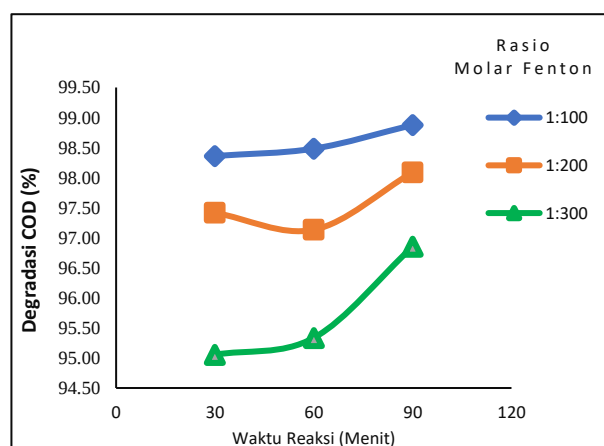
Gambar 3. Grafik Pengaruh Rasio Molar Fenton Dan Waktu Reaksi Terhadap Degradasi COD
