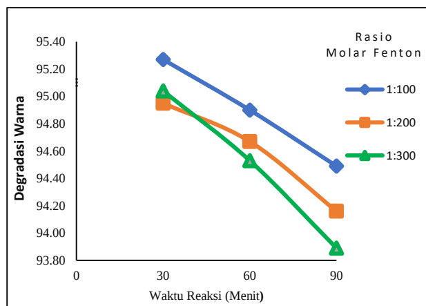
Gambar 2. Grafik Pengaruh Rasio Molar Fenton Dan Waktu Reaksi Terhadap Degradasi Warna
