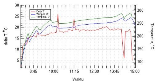
Gambar 2. Data Pengamatan Pemanasan Thermal Oil Menggunakan Pemanas Berbahan Bakar Solar Industri
