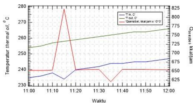
Gambar 3. Panas sensibel yang diperlukan untuk memanaskan thermal oil (11:00 – 12:00) WIB
