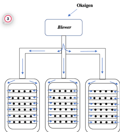
Gambar 1. Sistem aliran udara pada fine bubble diffuser
