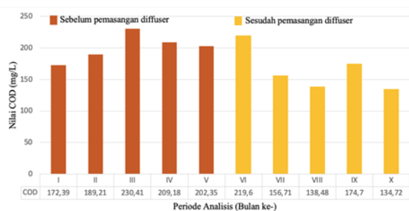
Gambar 3. Hasil analisis parameter COD limbah kolam aerobik sebelum dan sesudah pemasangan diffuser
