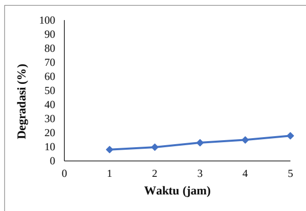
Gambar 10. Pagaruh waktu terhadap persentase degradasi methyl violet secara fotolisis
