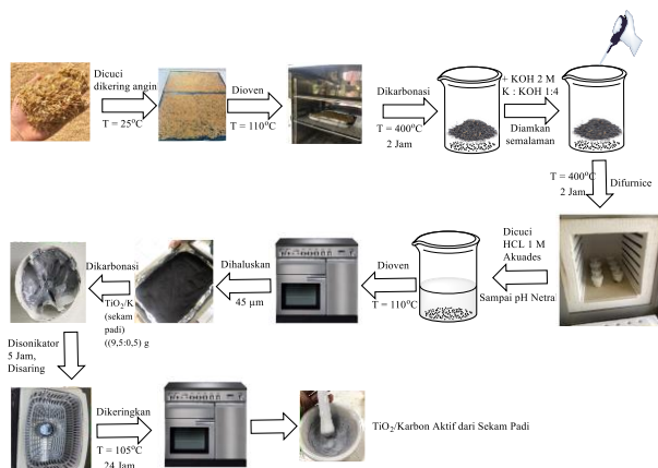
Gambar 1. Diagram skematik untuk preparasi TiO 2 /Karbon aktif dari sekam padi
