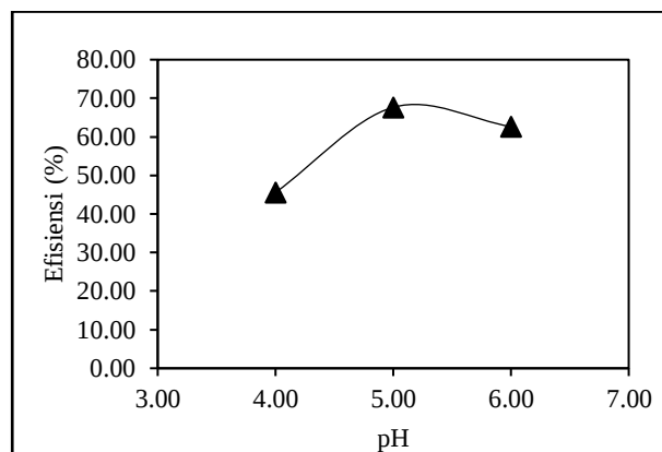
Gambar 4. Grafik hubungan antara pH larutan \text{Pb}^{2+} terhadap efisiensi adsorpsi
