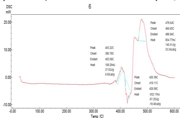
Gambar 5. Termoogram DSC Polistirena Tergrafting Maleat Anhidrida Sludge dan Abu Boiler 60:25:15
